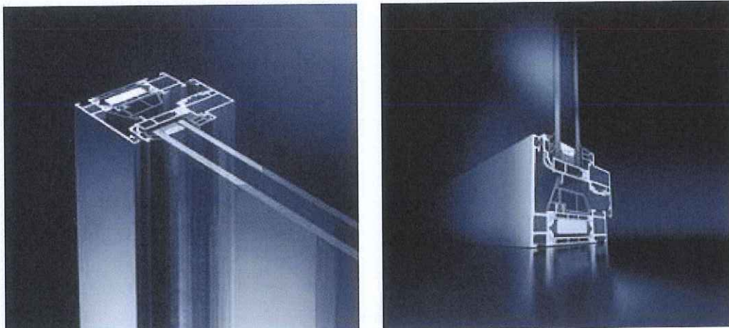
Genomskärning av fönster AWS 75BC.HI
